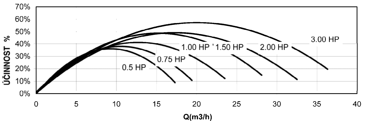
KŘIVKY ÚČINNOST - PRŮTOK
