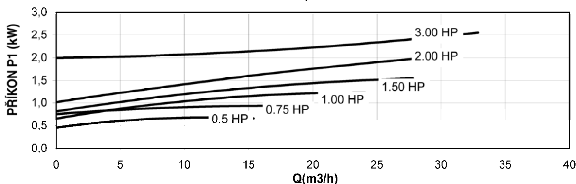
KŘIVKY PŘÍKON - PRŮTOK P1-Q
