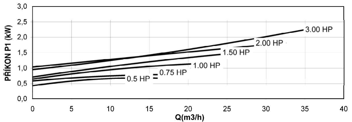
KŘIVKY PŘÍKON - PRŮTOK
